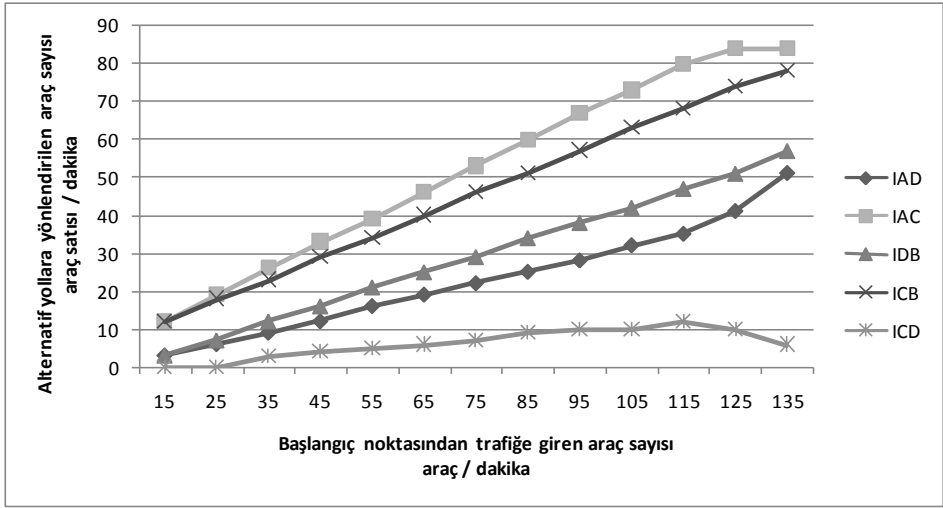
Şekil 2. Değişen trafik akışlarına göre alternatif hatların aldığı en iyi akış değerler grafiği
